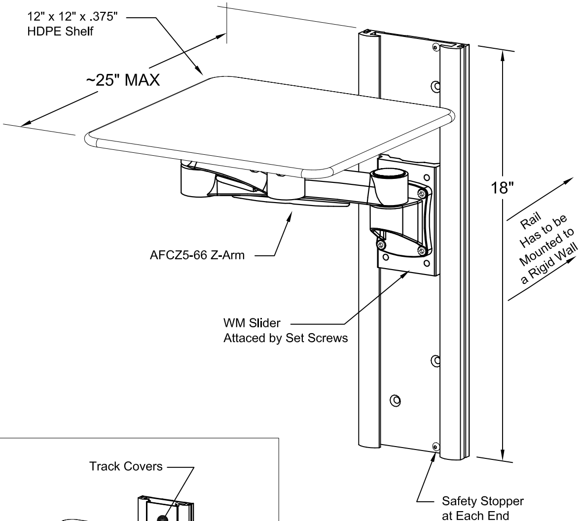
ISOMETRIC VIEW SCALE: ~3" = 1' - 0"
